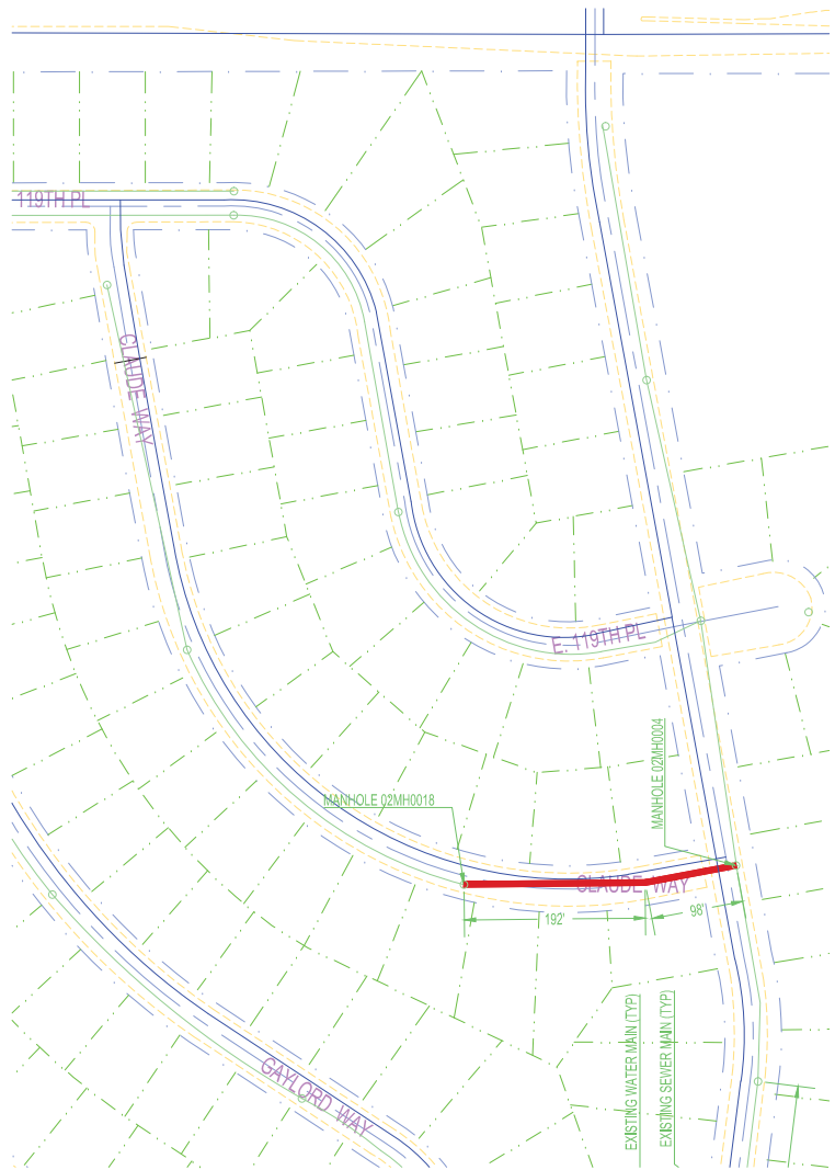
CLAUDE WAY 8" SANITARY SEWER N.T.S.
